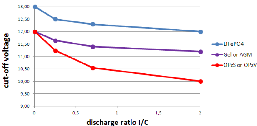
График соотношения разрядки и напряжения батареи для различных типов 12-вольтовых батарей (для 24 В умножьте на 2, а для 48 В умножьте на 4).
