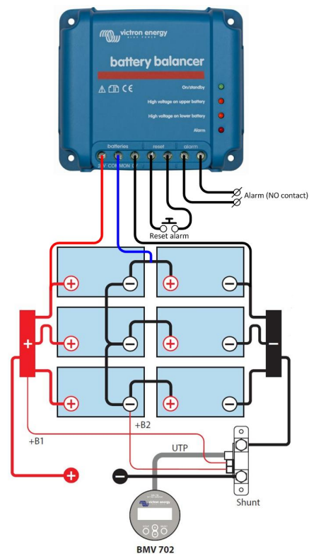
Battery Balancer, подключенный к шести последовательно-параллельно подключенным батареям на 12 В (24 В система)
